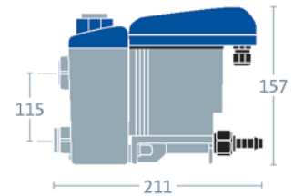
BEKOMAT 33 U
